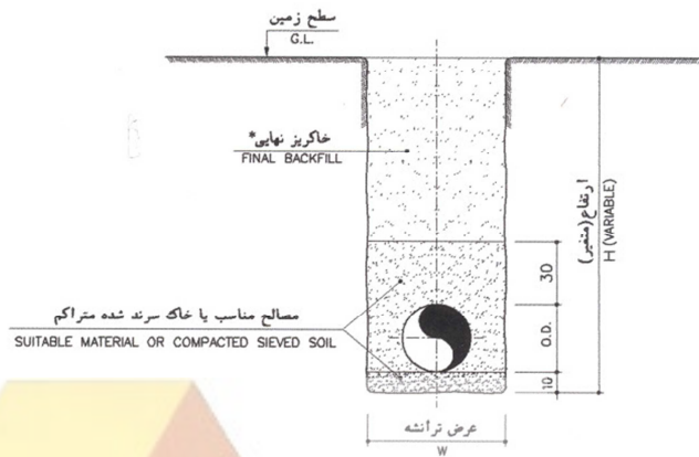
مقطع ترانشه
