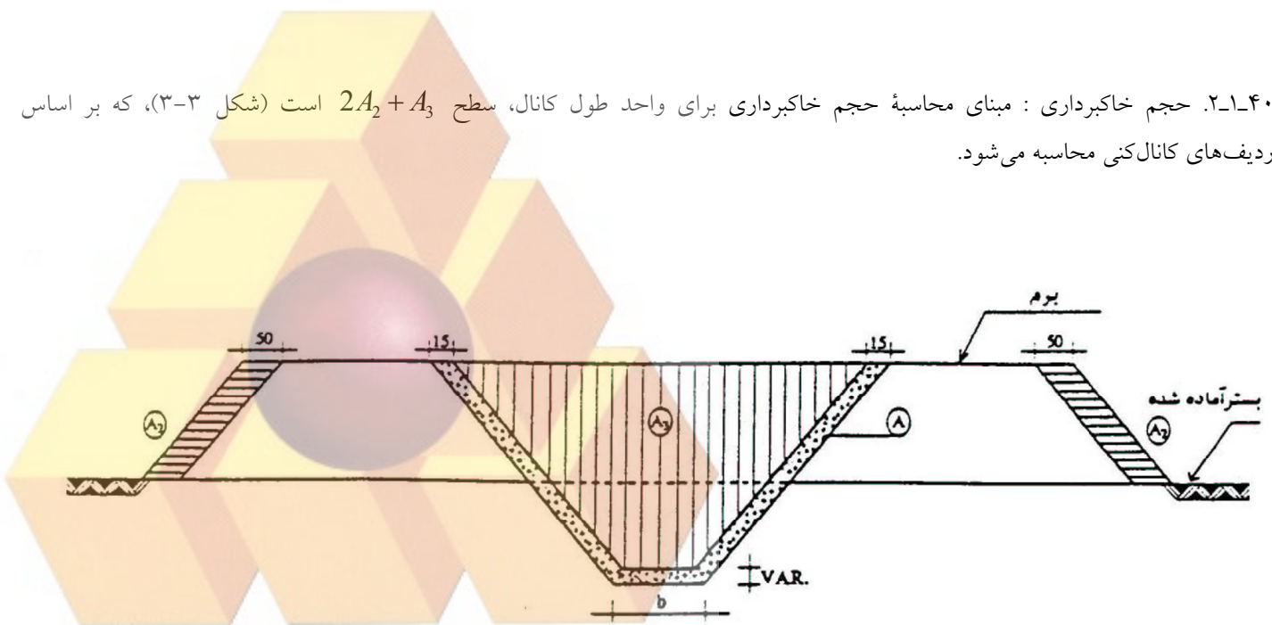
شکل ۳-۳. شمای مقطع خاکبرداری
